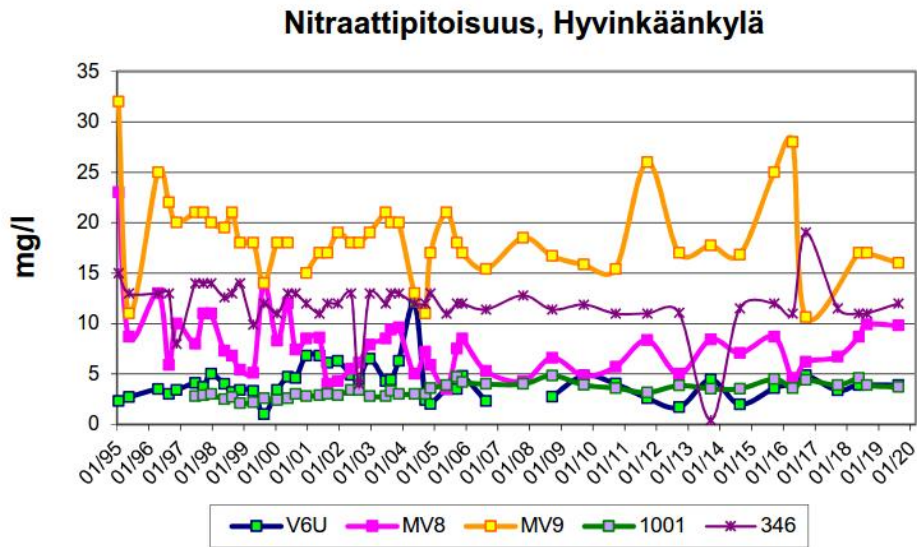
Kuva 5-2. Nitraattipitoisuuksien kehitys Hyvinkäänkylän tarkkailupisteissä V6U (aikaisemmin V6), MV8, MV9 ja 1001 (FCG, 2019).
