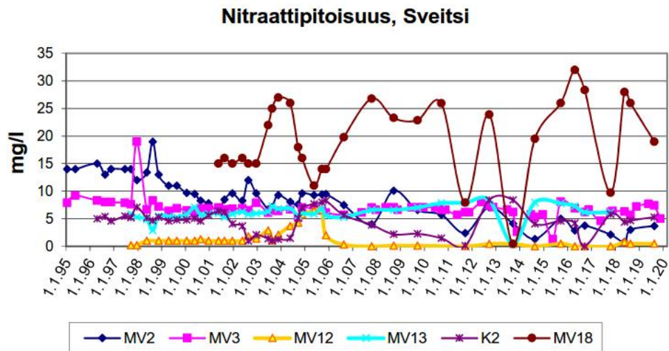
Kuva 5-4. Nitraattipitoisuuksien kehitys Sveitsin alueen tarkkailupisteissä MV2, MV3, K2, MV12, MV13 ja MV18 (FCG, 2019).
