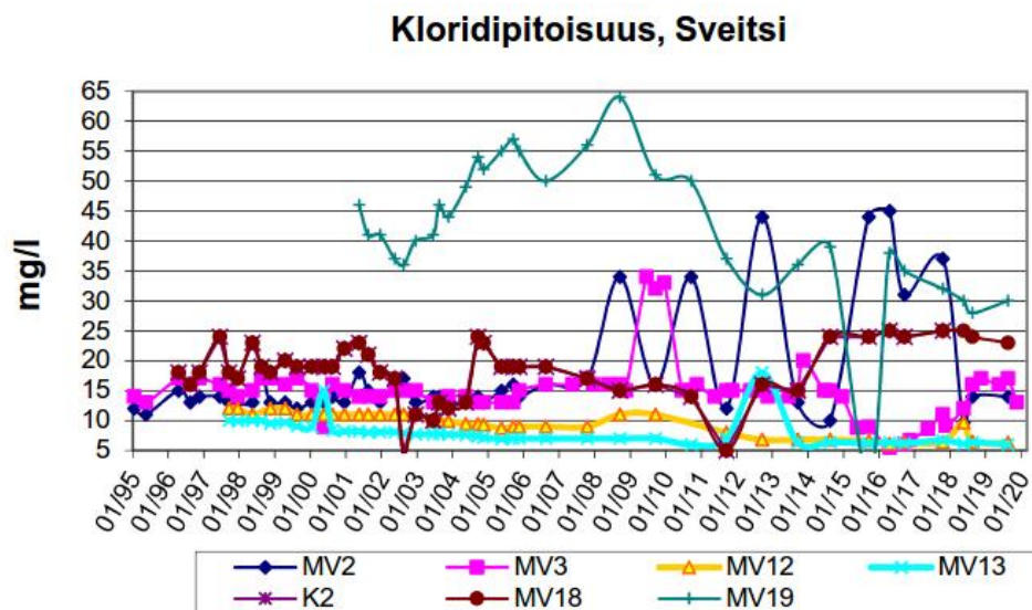
Kuva 5-3. Kloridipitoisuuksien kehitys Sveitsin alueen tarkkailupisteissä MV2, MV3, K2, MV12, MV13, MV18 ja MV19 (FCG, 2019).
