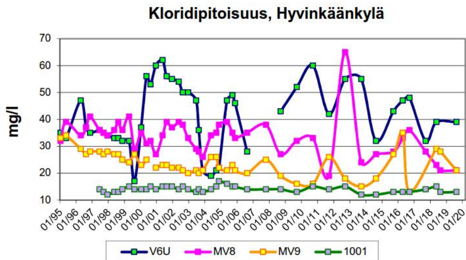
Kuva 5-1. Kloridipitoisuuksien kehitys Hyvinkäänkylän tarkkailupisteissä V6U (aikaisemmin V6), MV8, MV9 ja 1001 (FCG, 2019).
