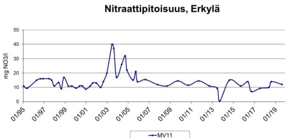
Kuva 5-5. Nitraattipitoisuuden kehitys Erkyliän tarkkailupisteessä MV11 (FCG, 2019).
